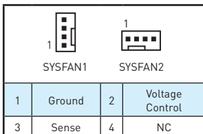
電壓模式風扇電源接頭
