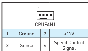
Connecteurs pour ventilateurs en mode PWM
