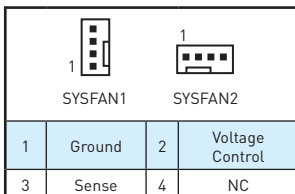
Connecteurs pour ventilateurs en mode tension
