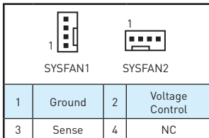
전압 모드 팬 커넥터
