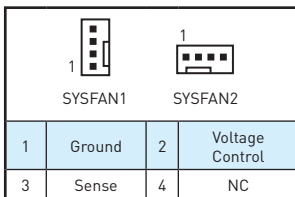
电压模式风扇接口
