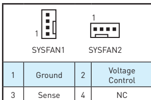
Lüfteranschluss des Spannung-Modus
