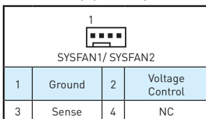
Разъем вентилятора режима напряжения
