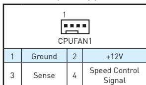
Разъем вентилятора с PWM управлением
