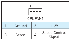
PWMモードファンコネクタ
