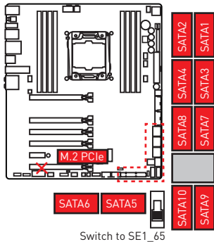
1xM.2 PCIe SSD + 10xSATA HDDs
