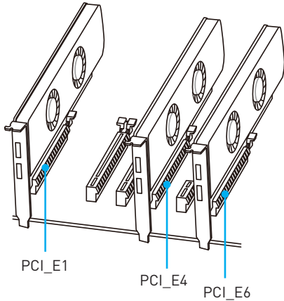
Pour les processeurs à 40 lignes
