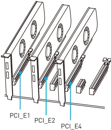
Pour les processeurs à 28 lignes
