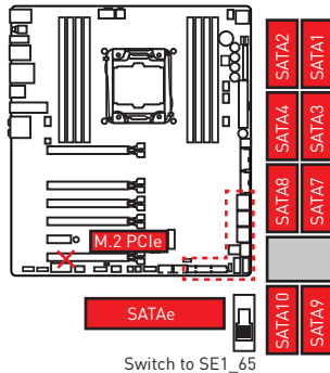
1xM.2 PCIe SSD + 8xSATA HDDs + 1xSATAe HDD
