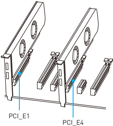
Pour les processeurs à 28 lignes
