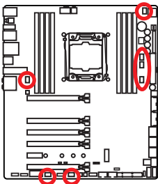
Voltage Mode fan connector
