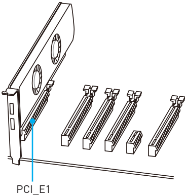
Pour les processeurs à 40 lignes
